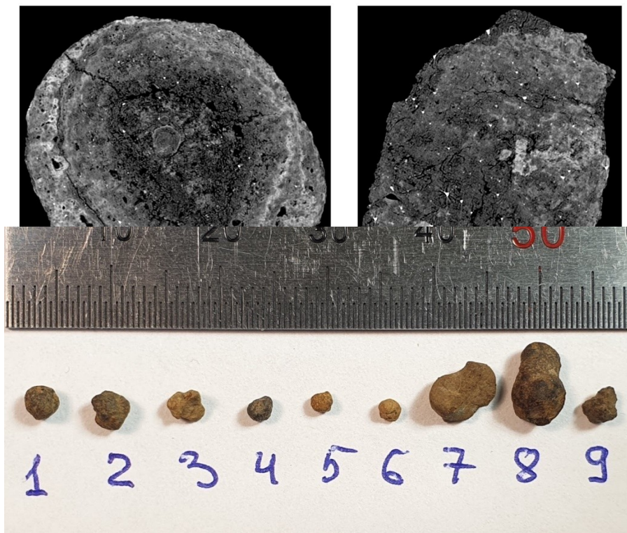
Рисунок 5 - Рентгеновские микротомограммы ортштейнов: а – фракция 1–2 мм; б – фракция 5–7 мм DOI: https://doi.org/10.60797/JAE.2026.74.2.5
