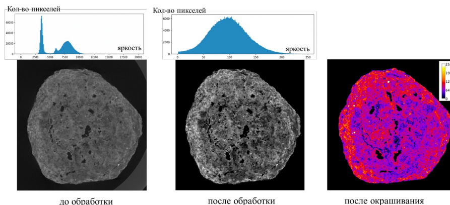
Рисунок 1 - Предобработка томографических изображений на примере томографического среза ортштейна 3-5 мм DOI: https://doi.org/10.60797/JAE.2026.74.2.1
